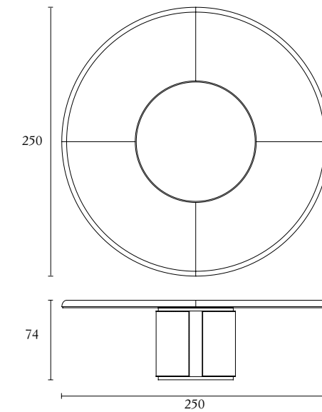
Cod. HELYTA250 cm Ø 250 x h 74 - inch 98.4 x 29.1
